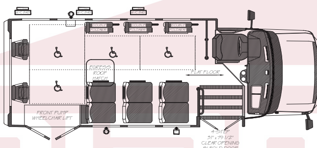
VIP 2200 - 6 PAS. & 4 W/C
